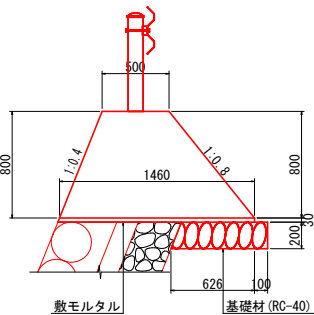
2号天端コンクリート
