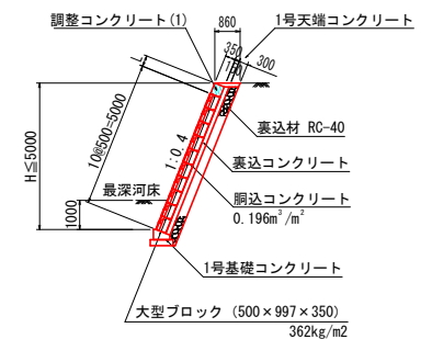
標準断面図 S=1/100
