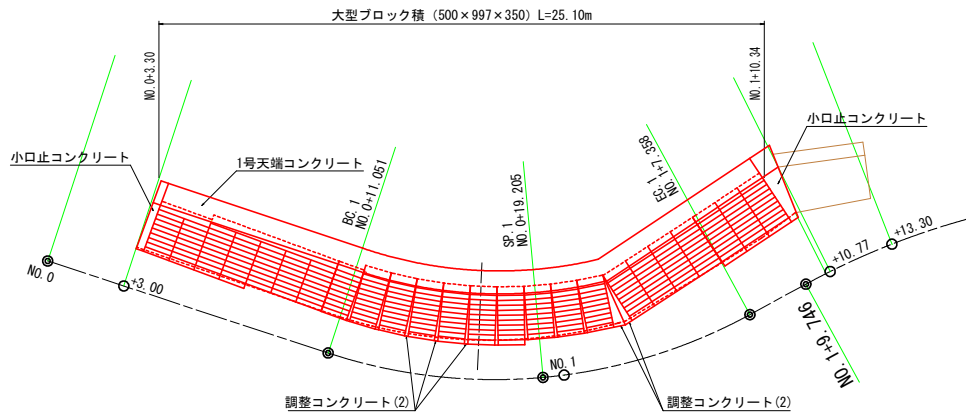
平面図 S=1/100
