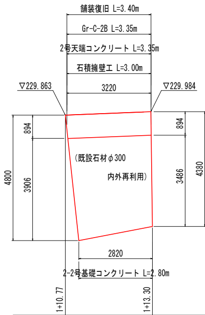
正面図
