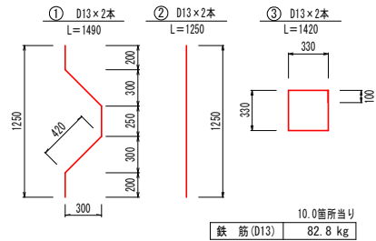
実施設計図面
