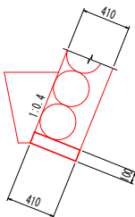
2-2号基礎コンクリート
