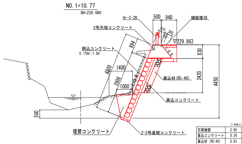
断面図
