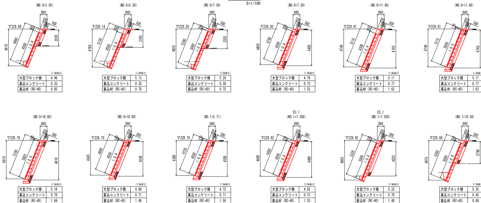
断面図 S=1/100
