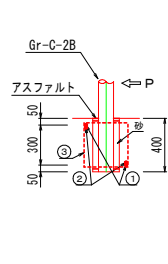
ガードレール補強鉄筋
